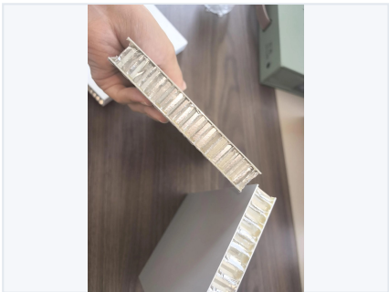
铝蜂窝板——防水、防潮、耐候，颜色可按客户要求定制。
