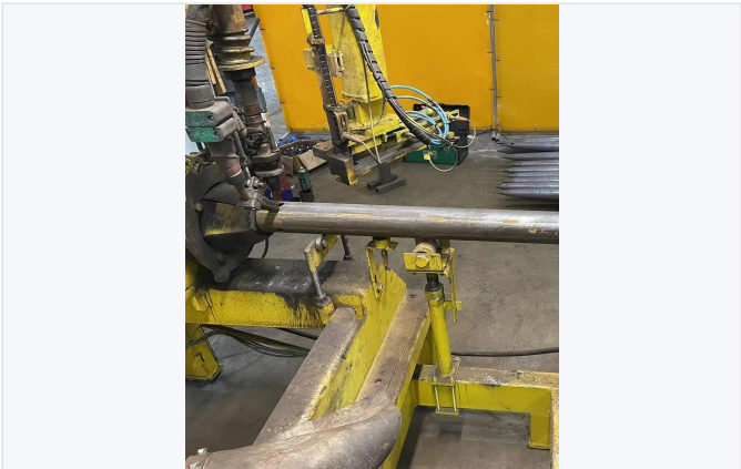
螺母焊接机——把螺母焊接至钢管上
