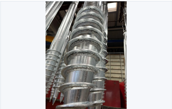
焊缝偏离钢管，导致钢带焊接不稳固且镀锌质量差
